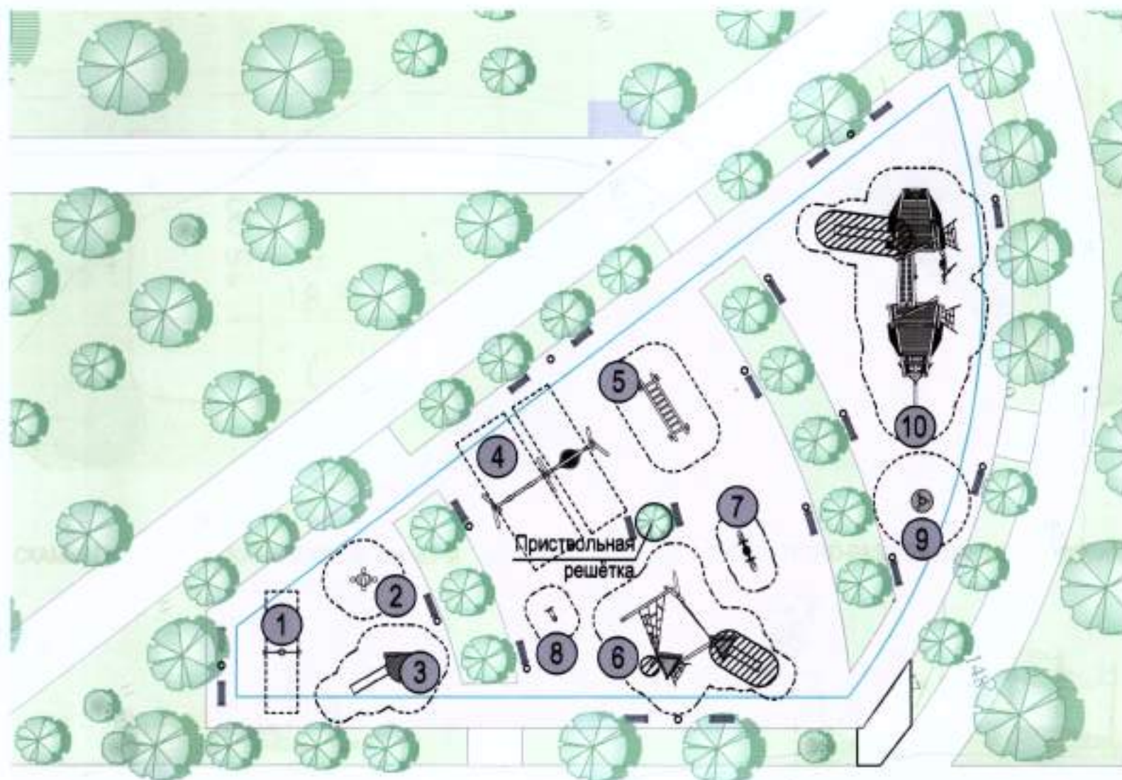
1 Качеля для детей от 1 до 3 лет (NRO902)
